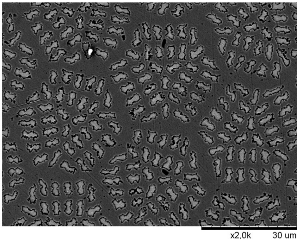
Рис. 2. Электронномикроскопическое изображения композиционных сверхпроводников.
