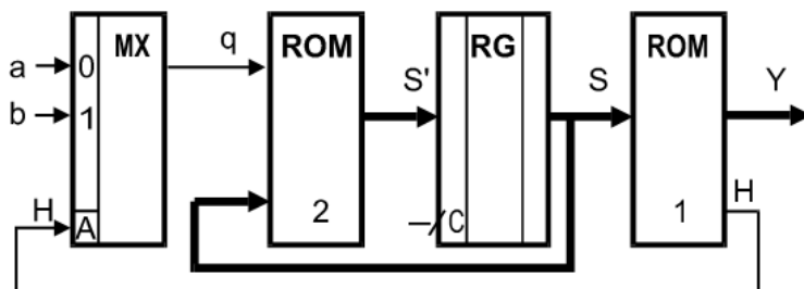
Рис.3. УА с адресным ПЗУ; последовательный вариант
