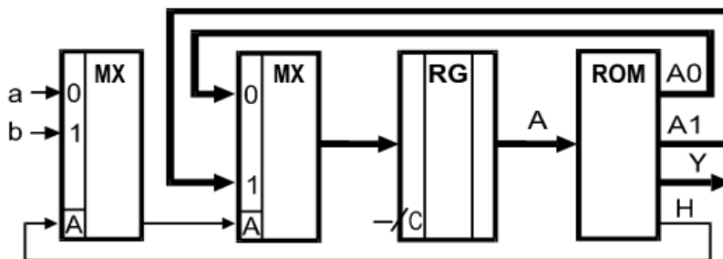
Рис.4. УА с явным указанием альтернативных адресов
