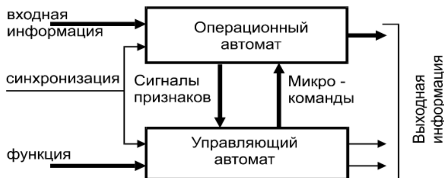
Рис.1. Структура вычислителя
